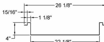
B-B
